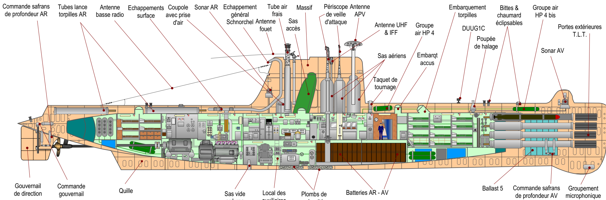
Coupe longitudinale après refonte
