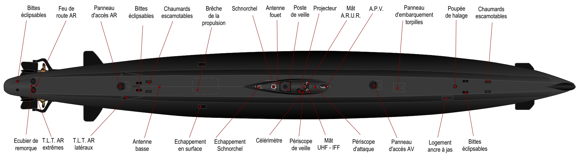
Vue de dessus au neuveage
