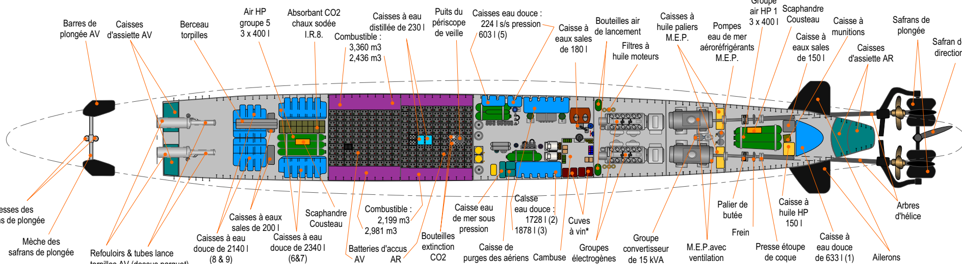
Coupe horizontale au-dessous du parquet au neuveage
