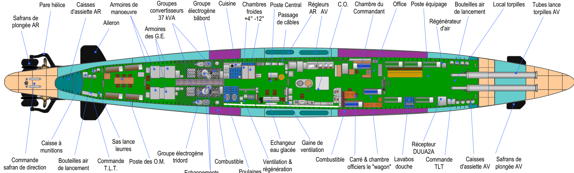
Coupe horizontale au-dessus du parquet
