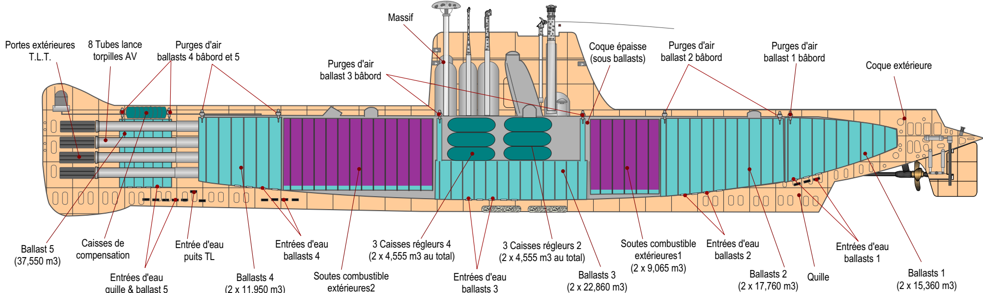
Coupe longitudinale partielle pour vue des ballasts au neuveage
