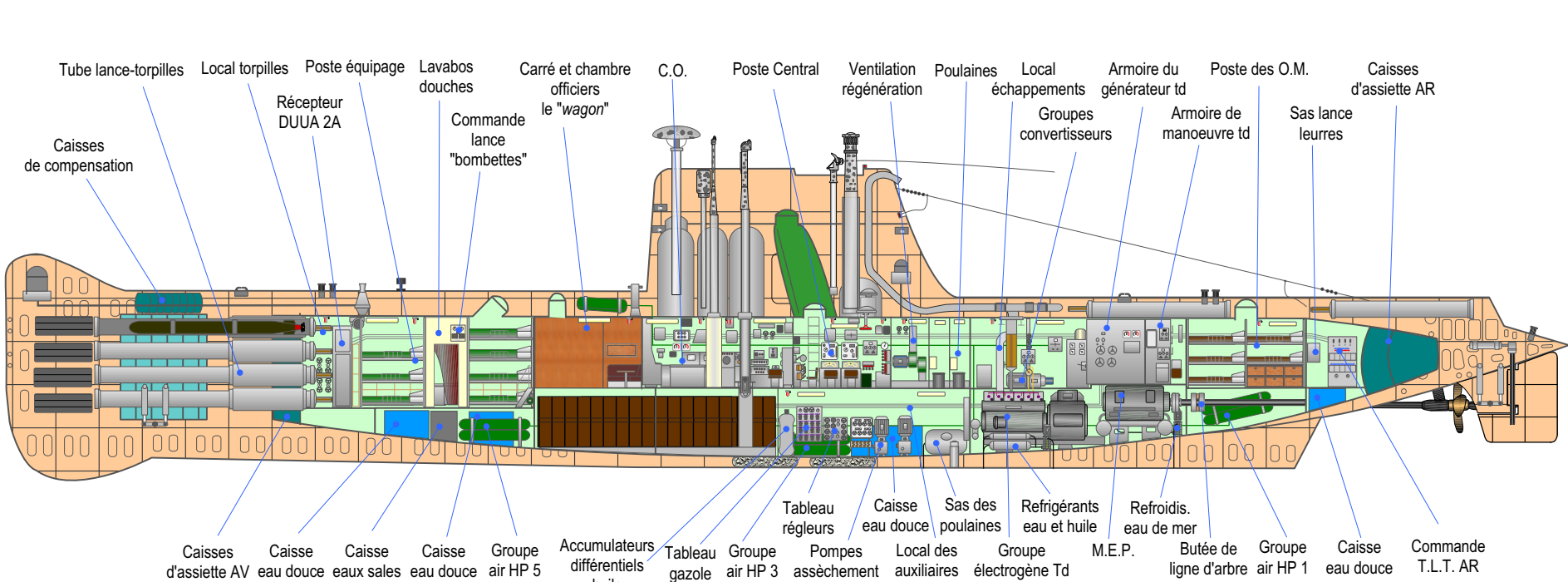
Coupe longitudinale au neuveage
