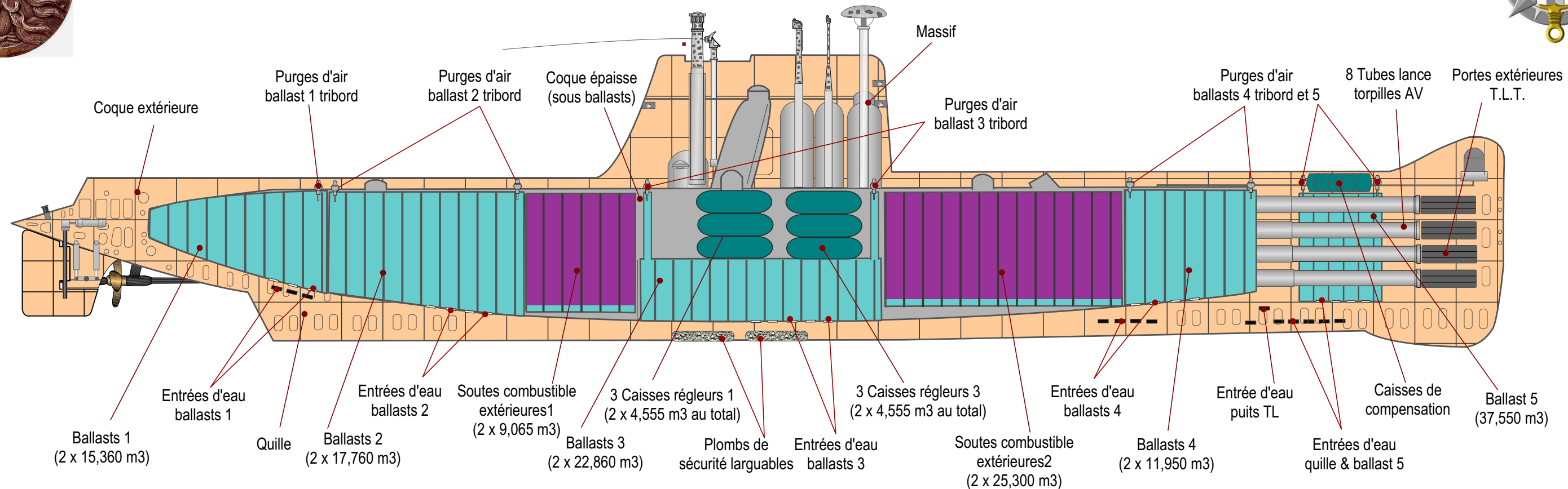
Coupe longitudinale partielle pour vue des ballasts au neuve
