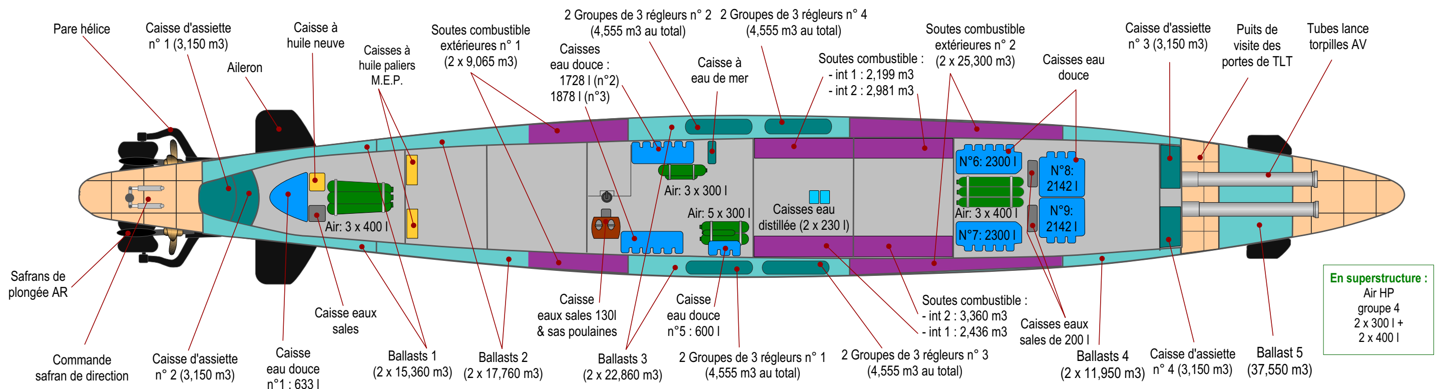
Coupe horizontale partielle au-dessous du parquet
