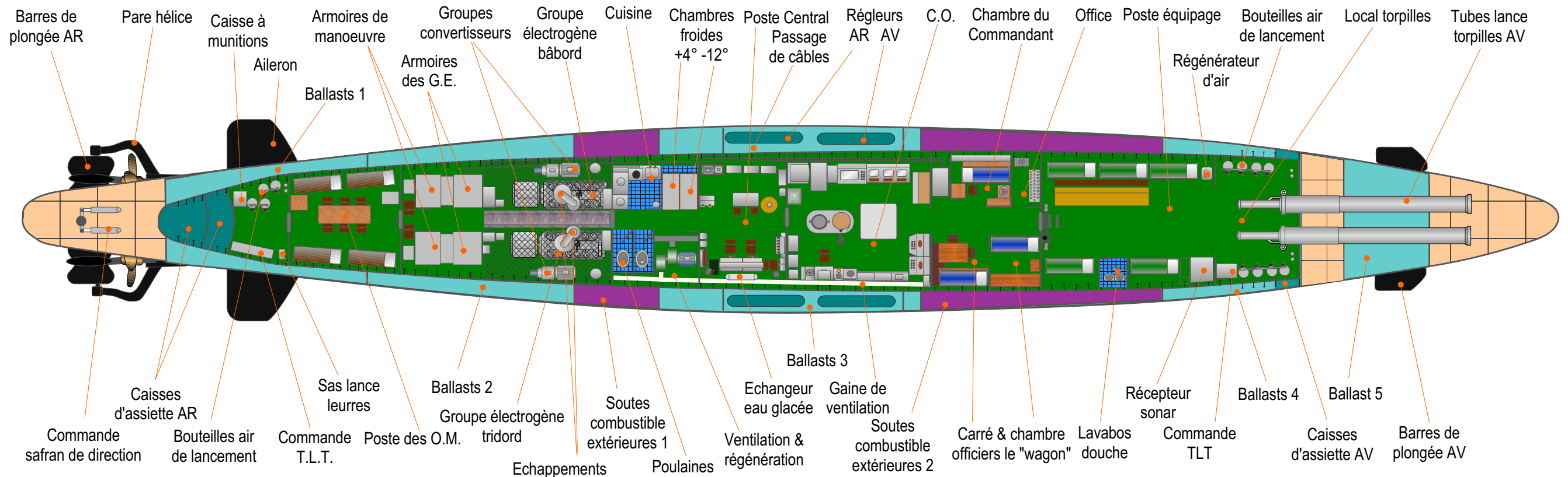
Coupe horizontale au-dessus du parquet
